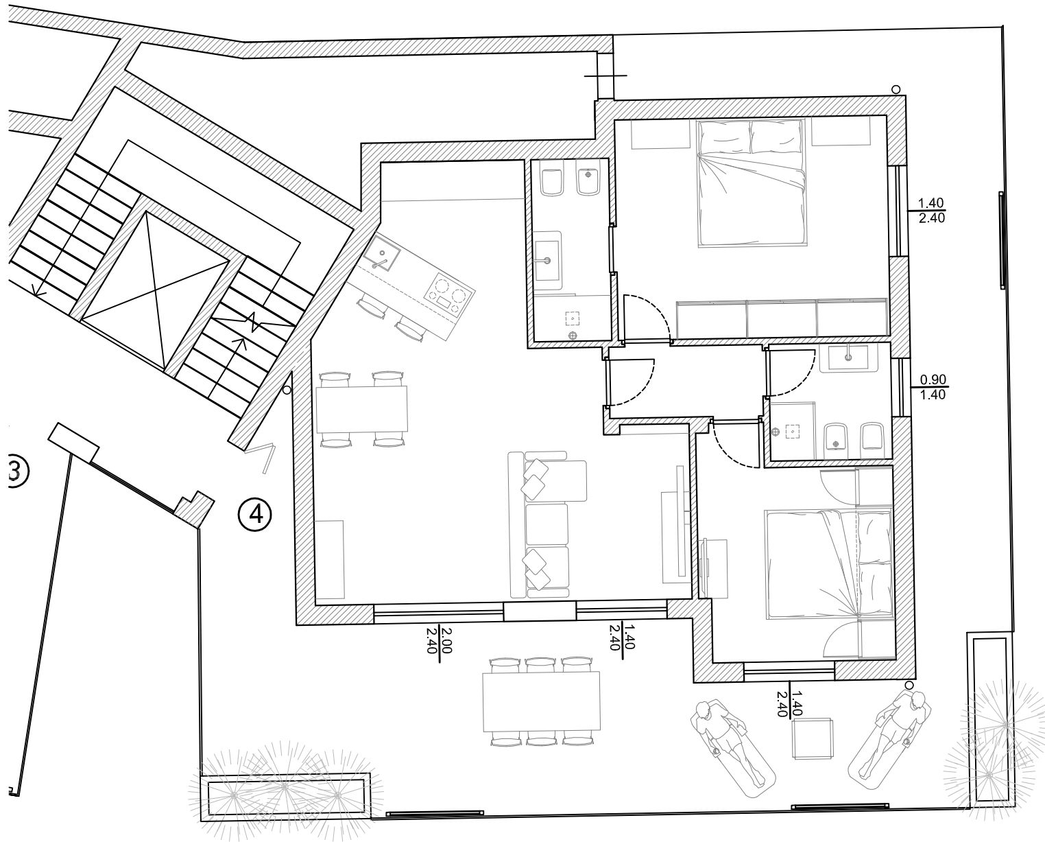
PIANO PRIMO
